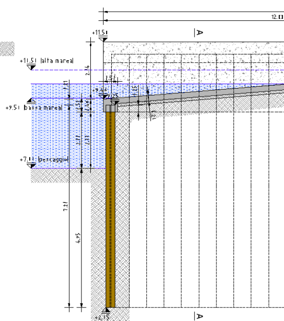
Sezione laterale scivolo
