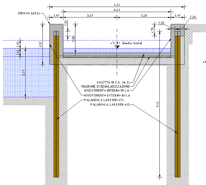
Sezione frontale scivolo
