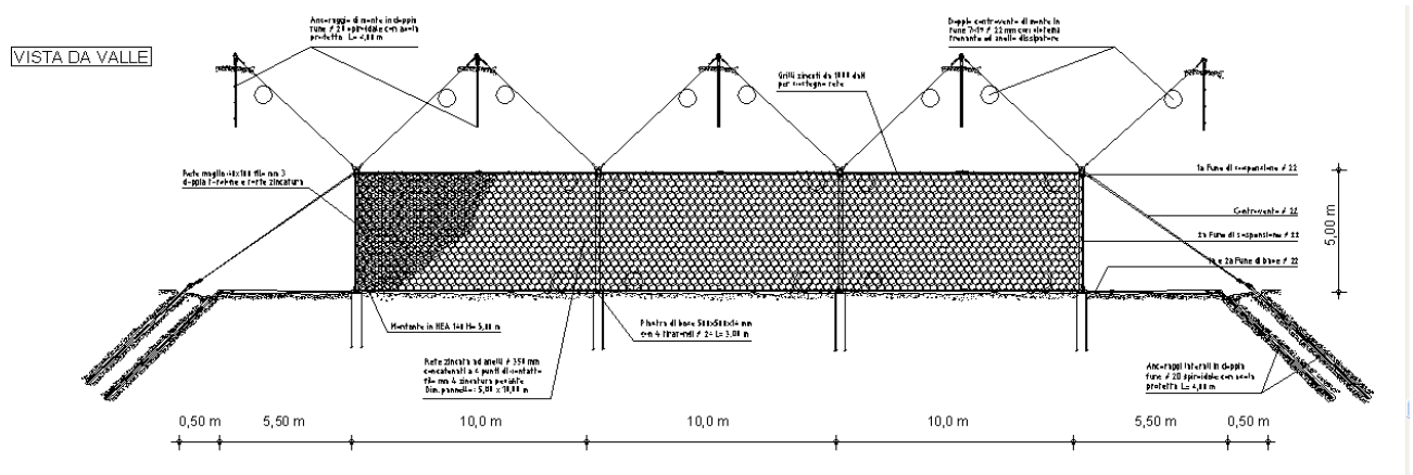
Schema strutturale
