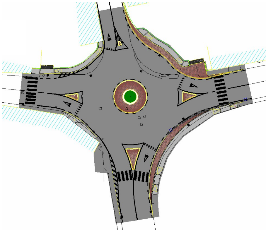
Planimetria di Progetto
