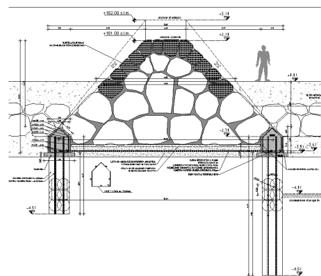
Sezioni di progetto dell'opera
