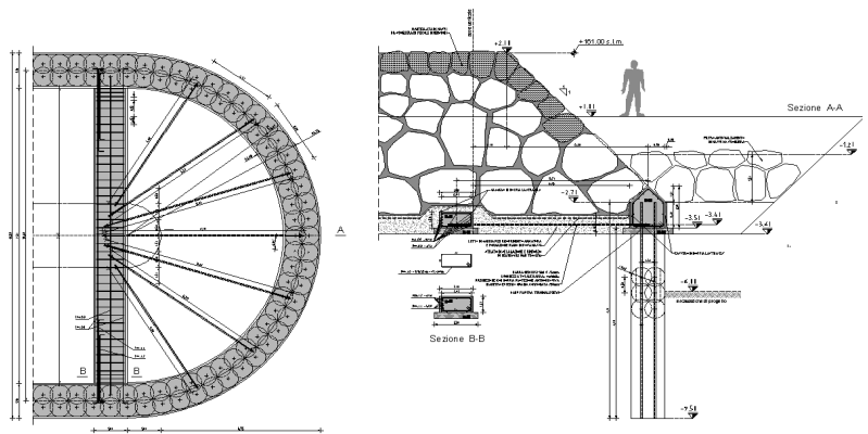
Sezioni di progetto dell'opera
