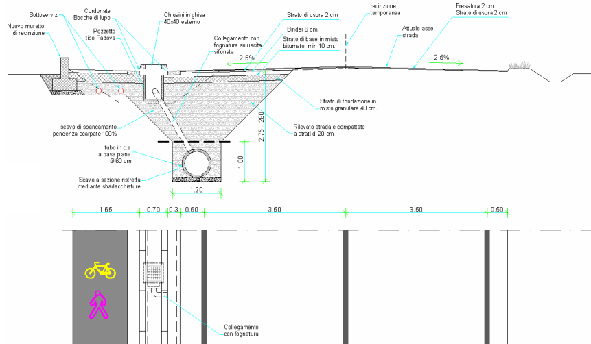
Sezione tipo via Matteotti
