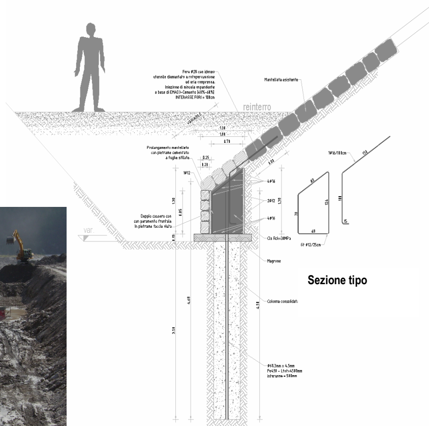
Rifacimento mantellata
