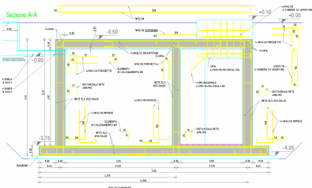
Sezione strutturale
