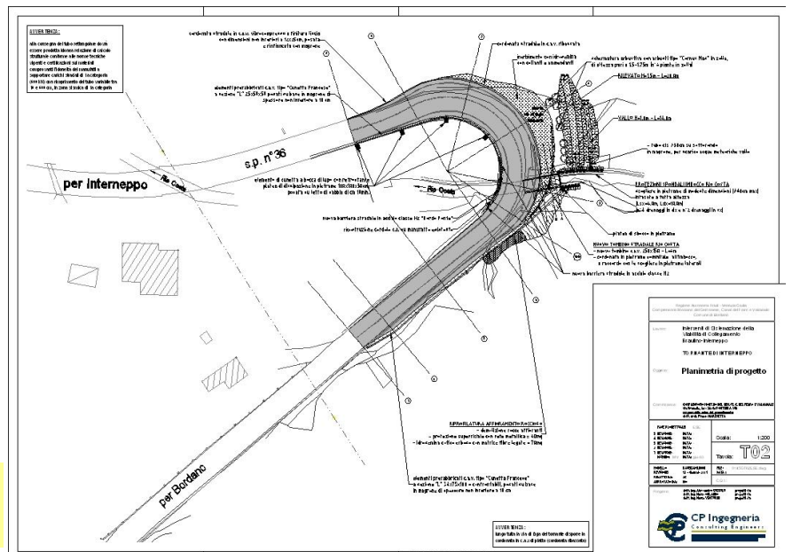
PLANIMETRIA DI PROGETTO “TORNANTE INTERNEPPO”
